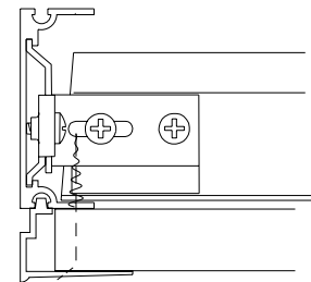
AXIOM de 2" con Borde Inferior de Mampostería sujeto al sistema de suspensión utilizando Abrazadera de Conexión a Perfil T
