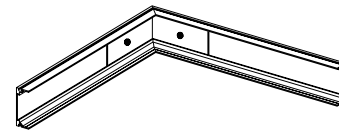
Junta a inglete cortada en fábrica o en obra. Ensamblada en obra usando el empalme de placa doblado según el ángulo deseado
